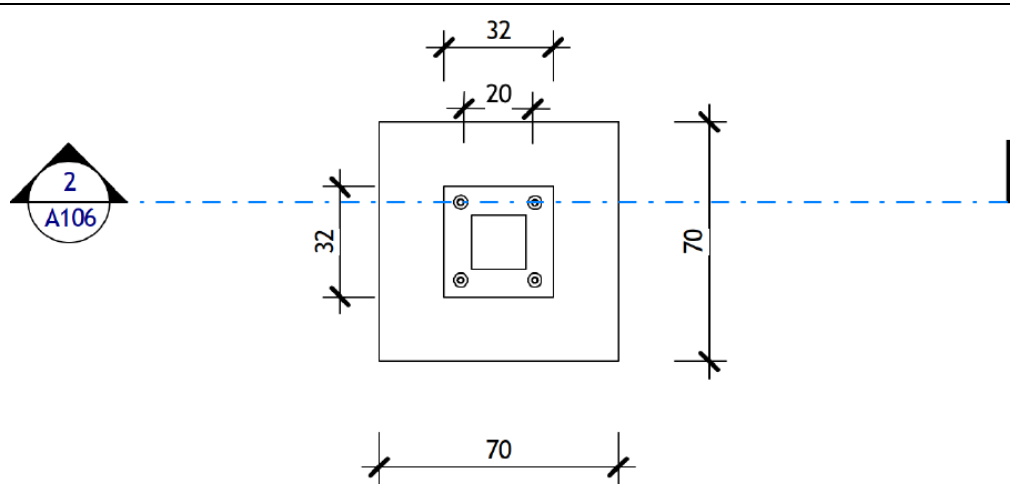
Detail massif de fondation
